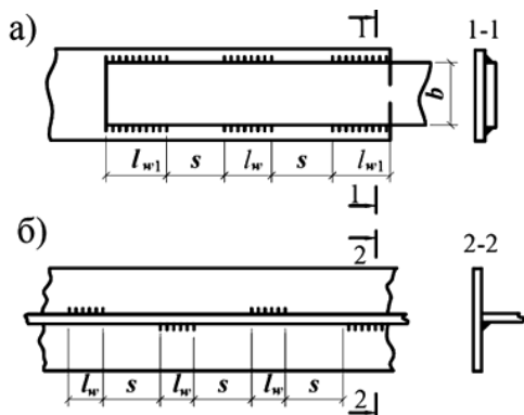
а - в нахлесточном соединении; б - в тавровом соединении
