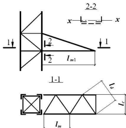
Рисунок 22 - Схема траверсы с треугольной решеткой
